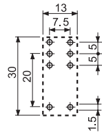
95.15.2 Вид сбоку
