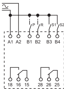
Схема подключения
